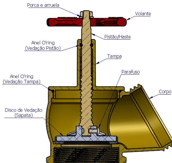
SEÇÃO A-A
