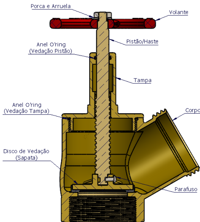
SEÇÃO A-A
